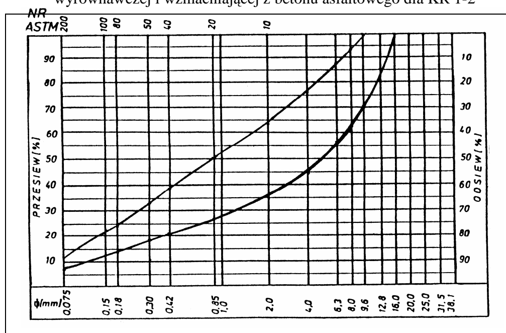
Rys. 1. Krzywe graniczne uziarnienia mieszanki mineralnej 0+16 mm do warstwy wiążącej, wyrównawczej i wzmacniającej z betonu asfaltowego dla KR 1-2
