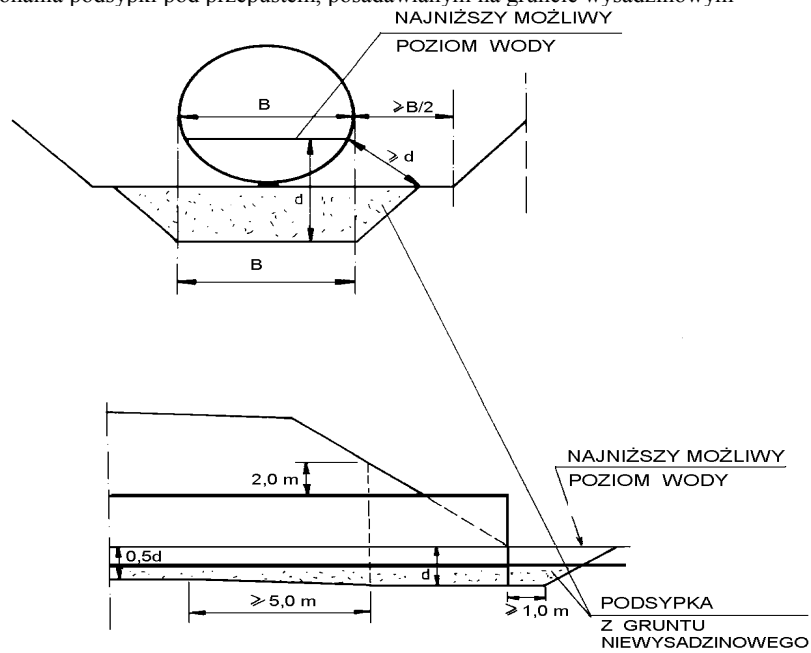
Rys. 6. Sposób wykonania podsypki pod przepustem, posadawianym na gruncie wysadzinowym
