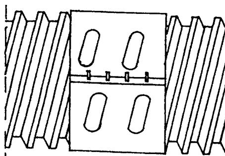
Rys. 3. Dwa odcinki rur połączone złączką zaciskową z blachy stalowej grubości 3 mm ocynkowanej galwanicznie (Istnieją również złączki plastikowe)
